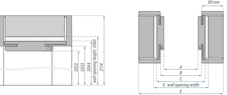
ADJUSTABLE 80 DOOR FRAME ADJUSTABLE 80 DOOR FRAME
