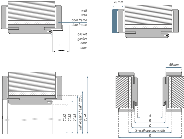
ADJUSTABLE DOOR FRAME ADJUSTABLE DOOR FRAME
